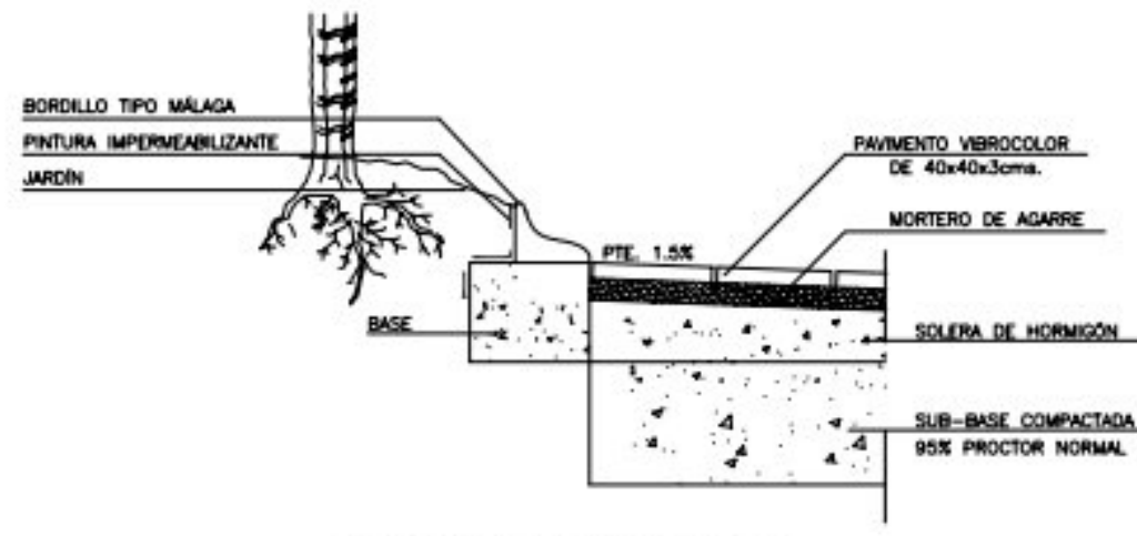
DETALLE DE BORDILLO PARTERRE
