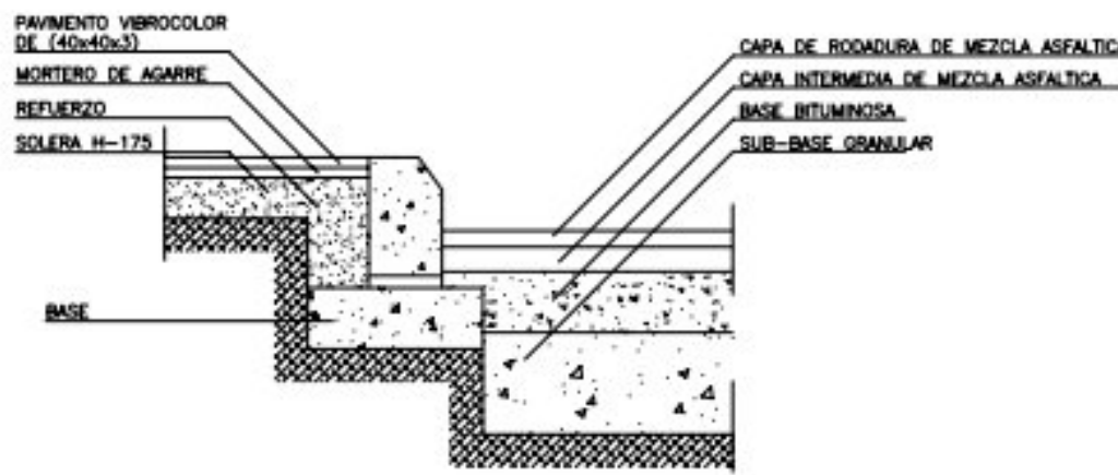
DETALLE DE BORDILLO
